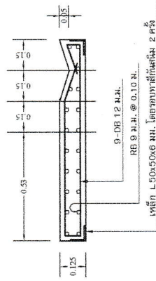
รูปตัดขยายคาน้ำปัดน้ำทิ้ง ขนาดพื้นที่ 1:25
